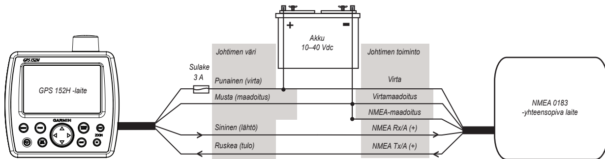
GPS 152H -laitteen liittäminen Standard NMEA 0183 -laitteeseen
